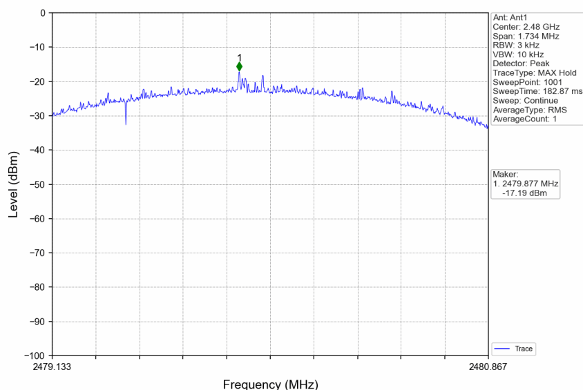
2M_HCH_2480MHz_DataRate=_Ant1_NTNV
