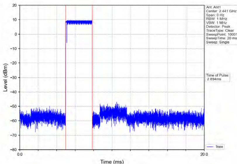
Pi/4DQPSK_2DH5_HOPP_Ant1_NTNV
