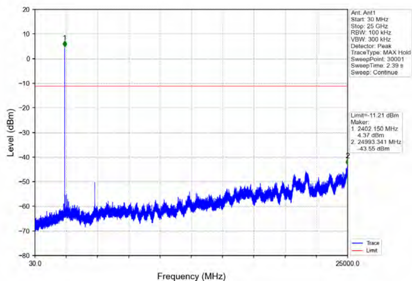
8DPSK 3DH5 LCH 2402MHz Ant1 NTNV
