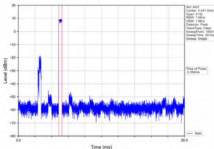
Pi/4DQPSK_2DH1_HOPP_Ant1_NTNV
