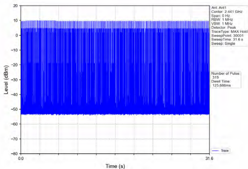
Pi/4DQPSK_2DH1_HOPP_Ant1_NTNV
