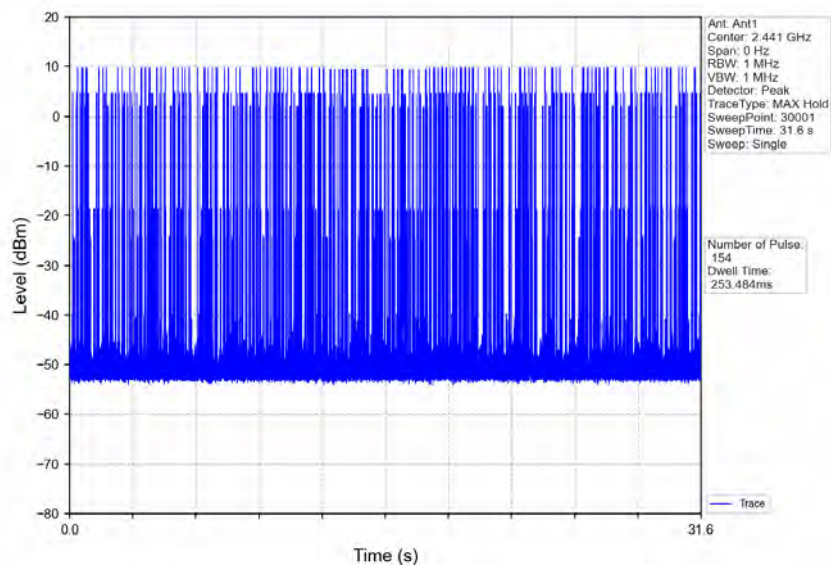
Pi/4DQPSK_2DH3_HOPP_Ant1_NTNV
