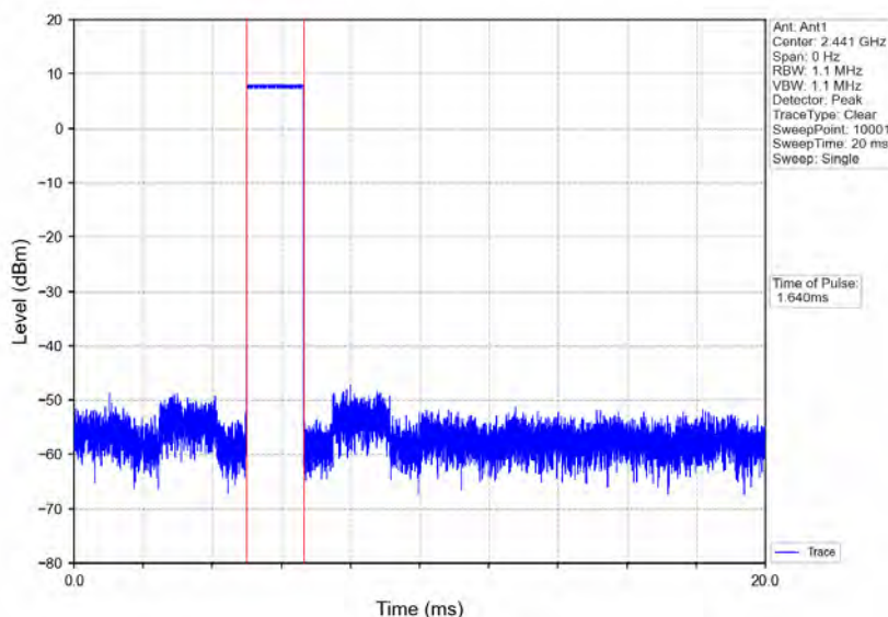
GFSK DH3 HOPP Ant1 NTNV
