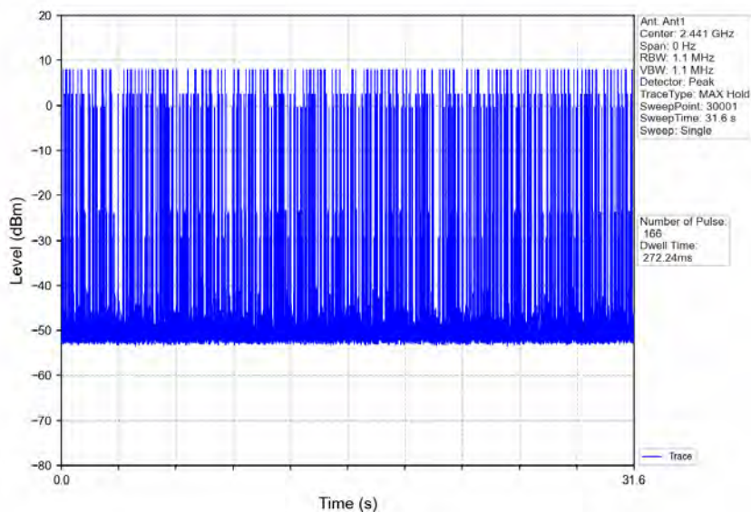
GFSK DH3 HOPP Ant1 NTNV
