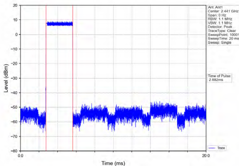
8DPSK_3DH5_HOPP_Ant1_NTNV
