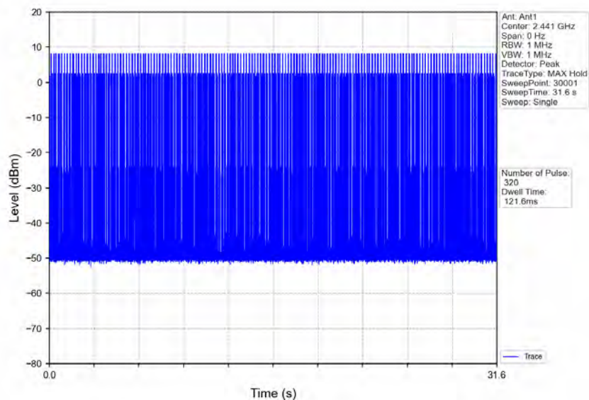
Pi/4DQPSK_2DH1_HOPP_Ant1_NTNV
