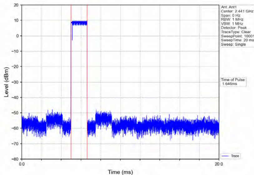
Pi/4DQPSK_2DH3_HOPP_Ant1_NTNV
