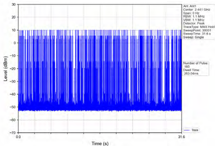
8DPSK_3DH3_HOPP_Ant1_NTNV
