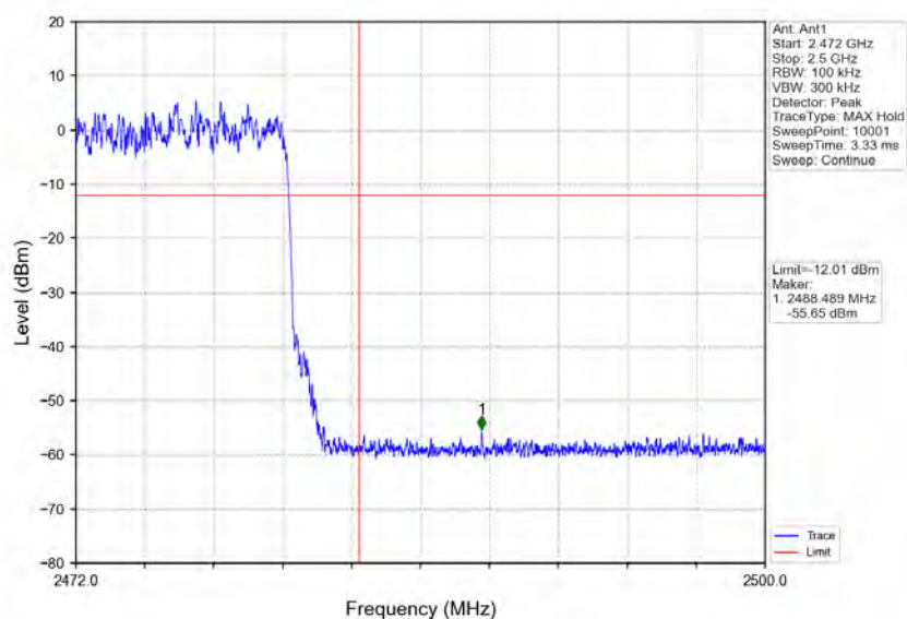
8DPSK_3DH5_HOPP_Ant1_NTNV
