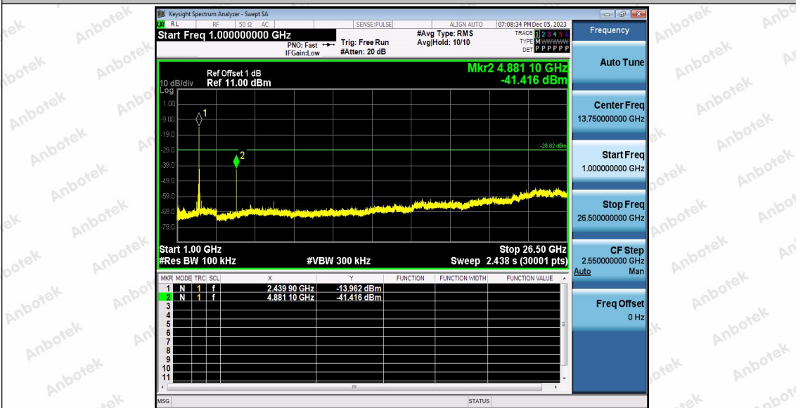
2.4G_Ant1_2440_1000~26500
