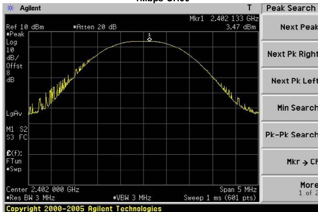
1Mbps-CH00
