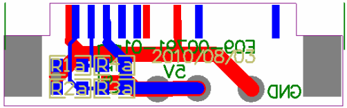
Connector PCB BOT
