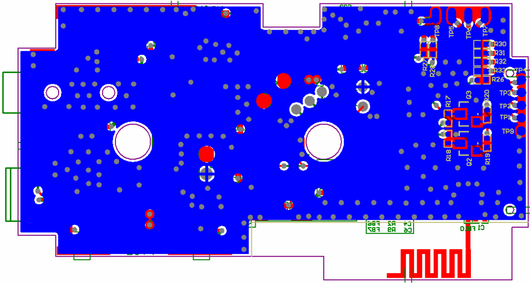
MAIN PCB BOT
