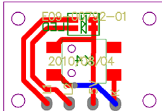
Button PCB BOT
