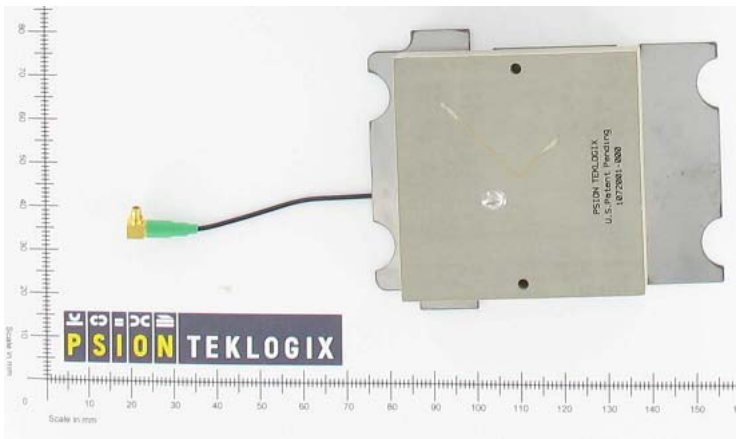
RFID MODULE UHF-CA3-AC5-XMOD: Antenna
