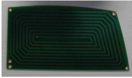
RFID MODULE HF-T2-G2: Assembly
