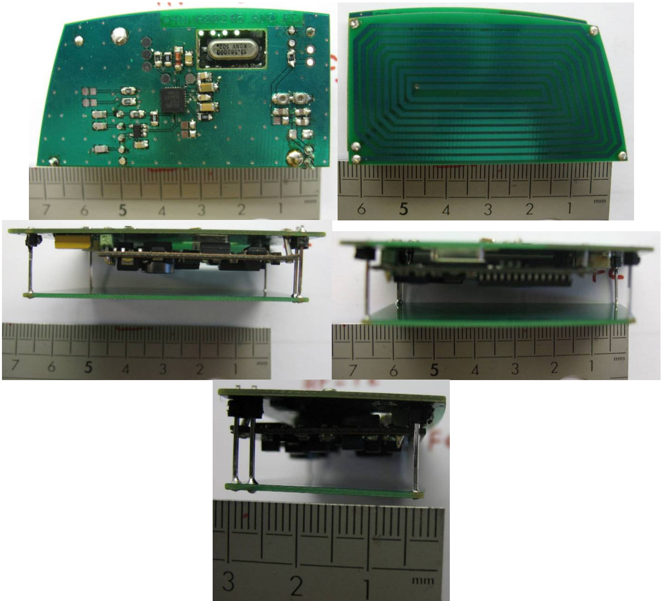
RFID MODULE HF-T2-G2: Assembly
