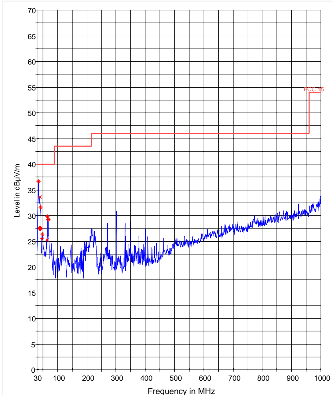
FCC 15 30-1000MHz
