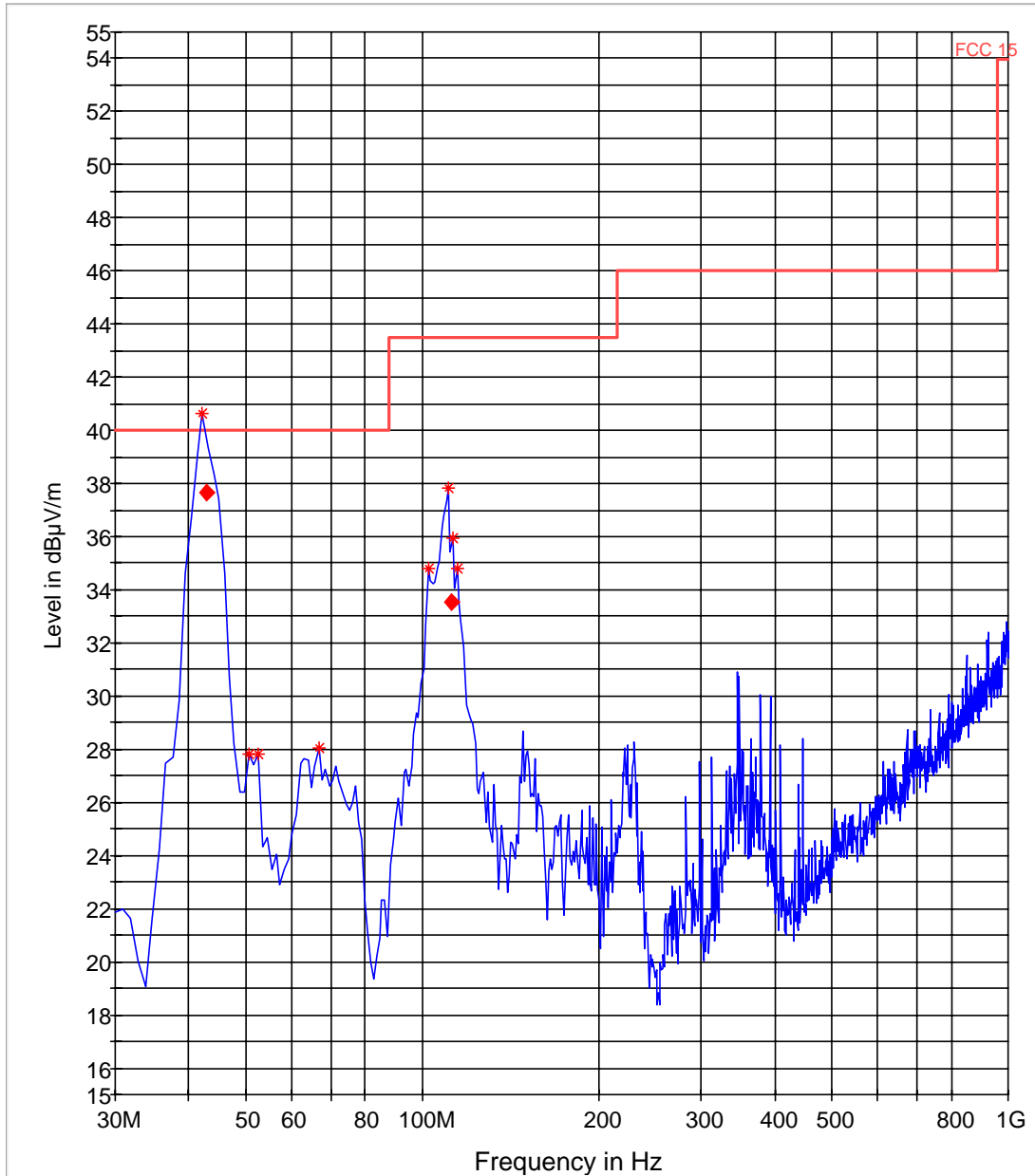
FCC 15 30-1000MHz
