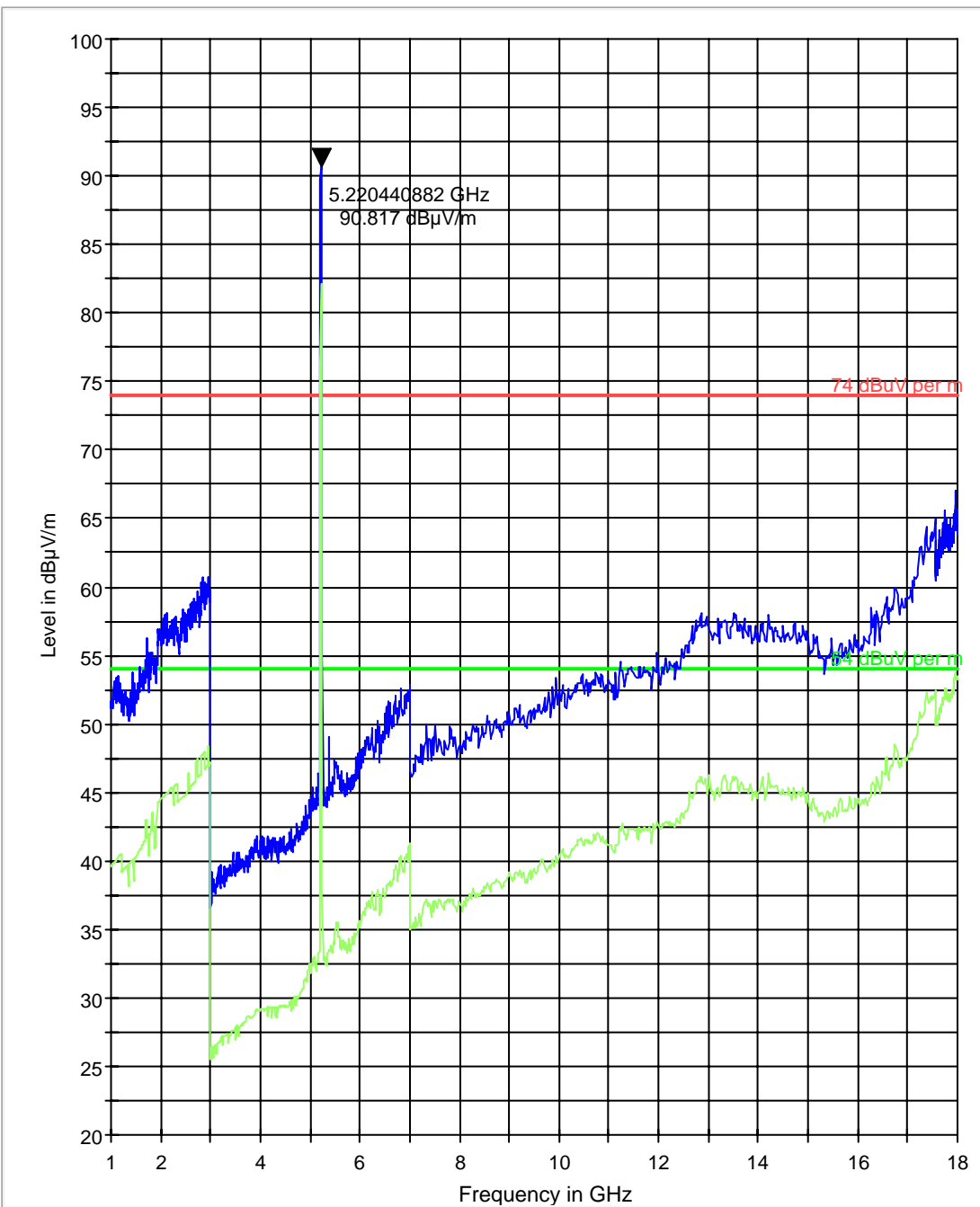
FCC 15 1-18GHz
