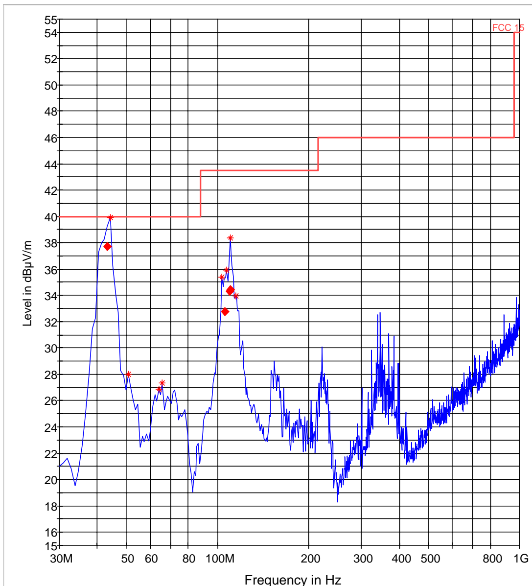
FCC 15 30-1000MHz
