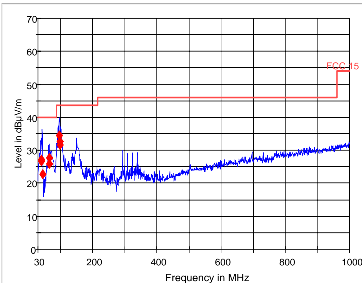
FCC 15 30-1000MHz
