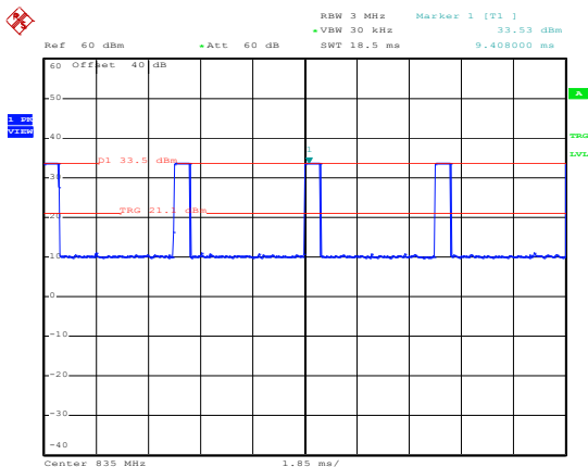
835MHz - GSM
