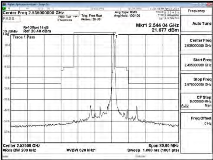
Band7_20MHz_16QAM_1_99_CH21350
