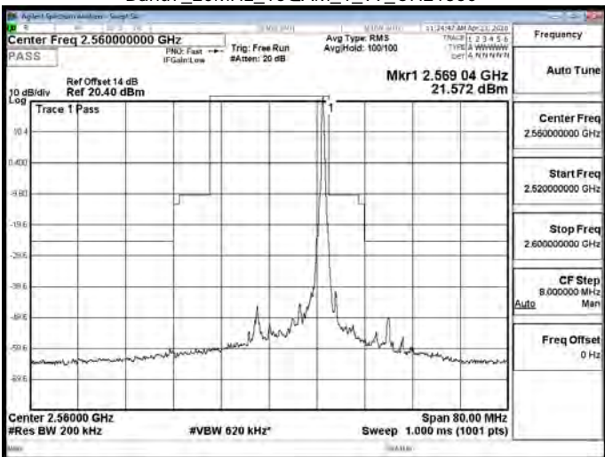
Band7_20MHz_16QAM_1_99_CH21350
