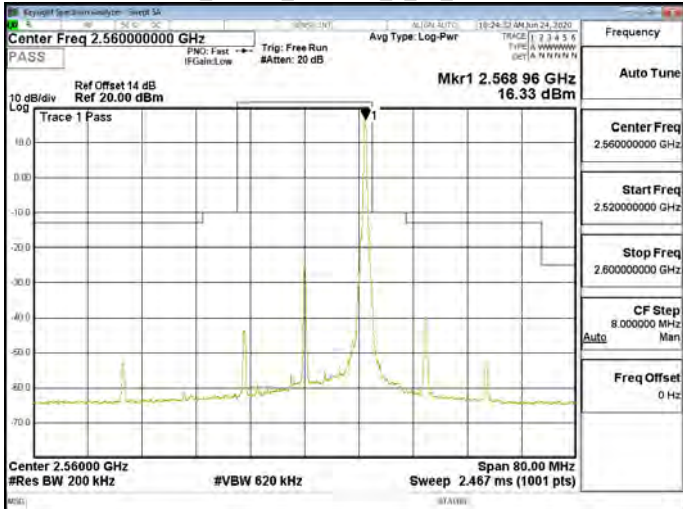
Band7_20MHz_256QAM_1_99_CH21350
