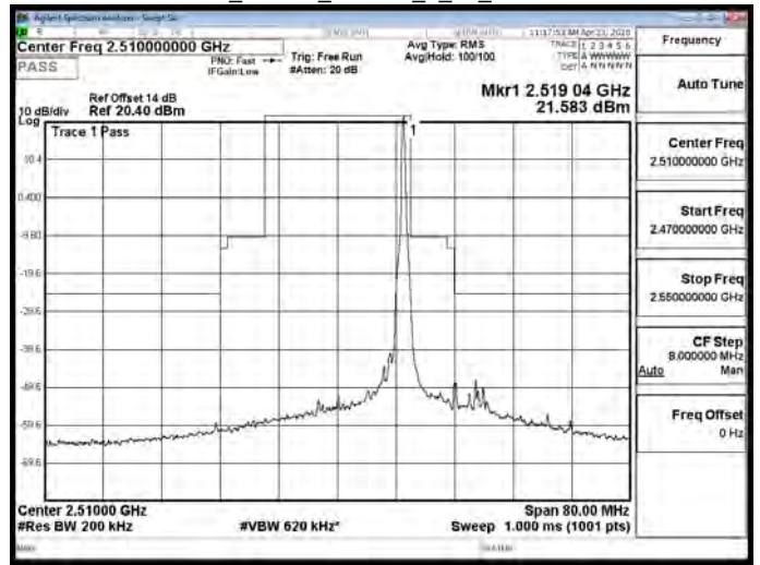
Band7_20MHz_64QAM_1_99_CH21100
