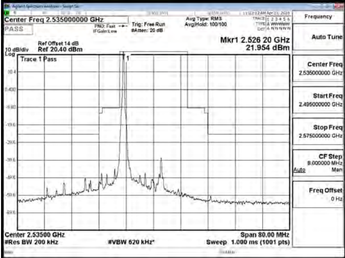
Band7_20MHz_QPSK_1_0_CH21350
