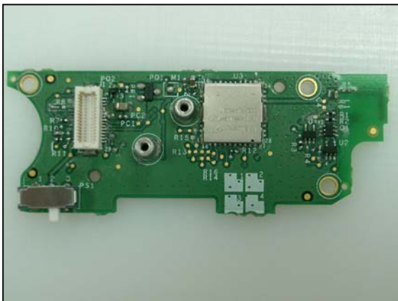
BT Ant.
