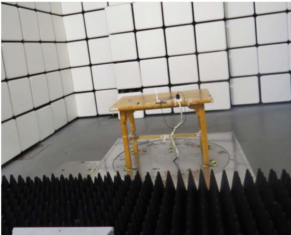
1GHz-18GHz
