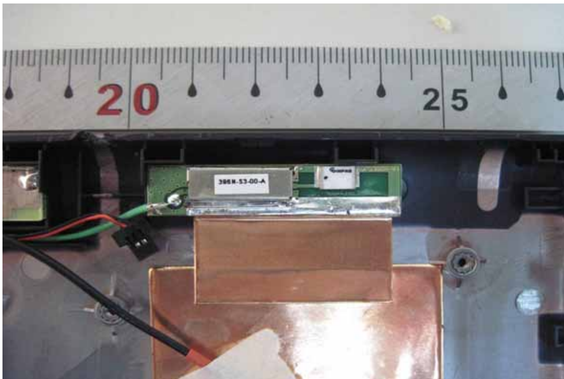
GPS Antenna
