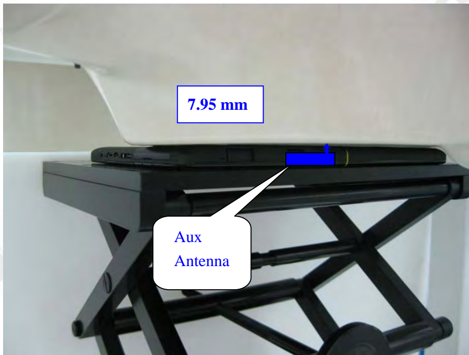
Fig.3.2 Lap-held mode (Aux antenna)
