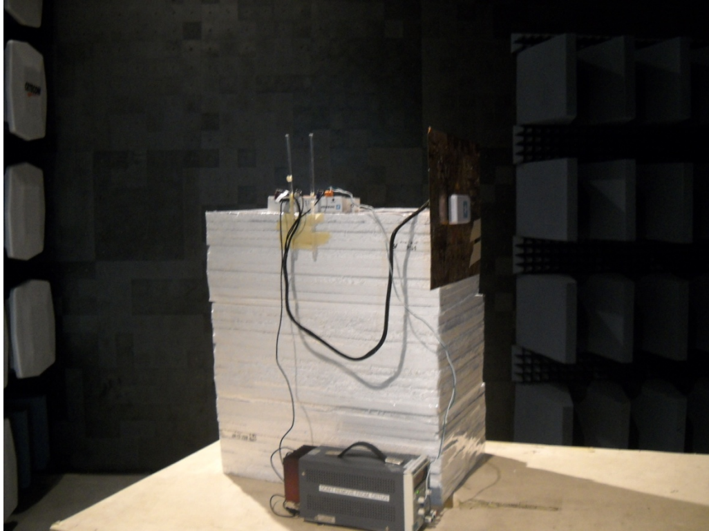
Fig. 1 EUT Setup
