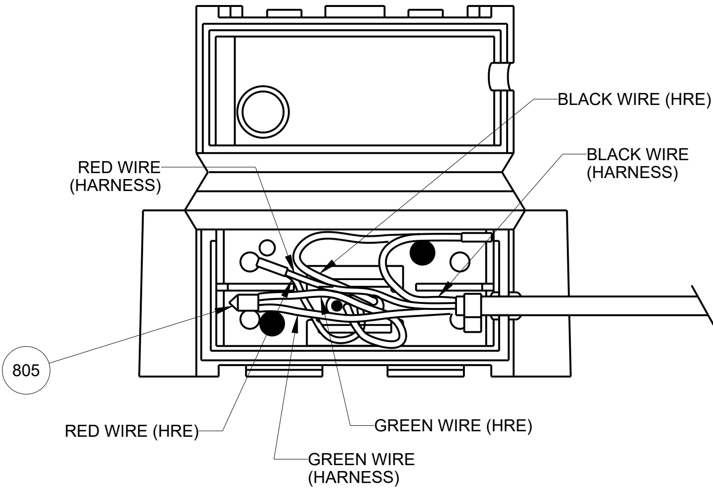
VIEW A-A SCALE: 2:1
