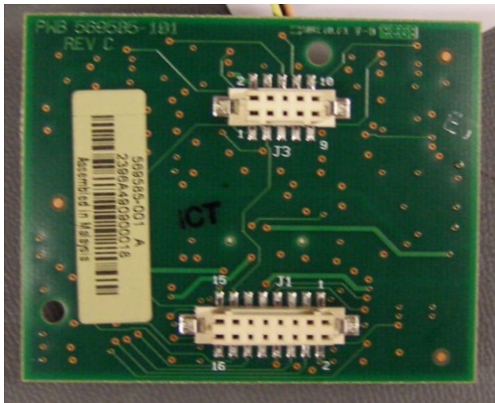
Mag Stripe Back
