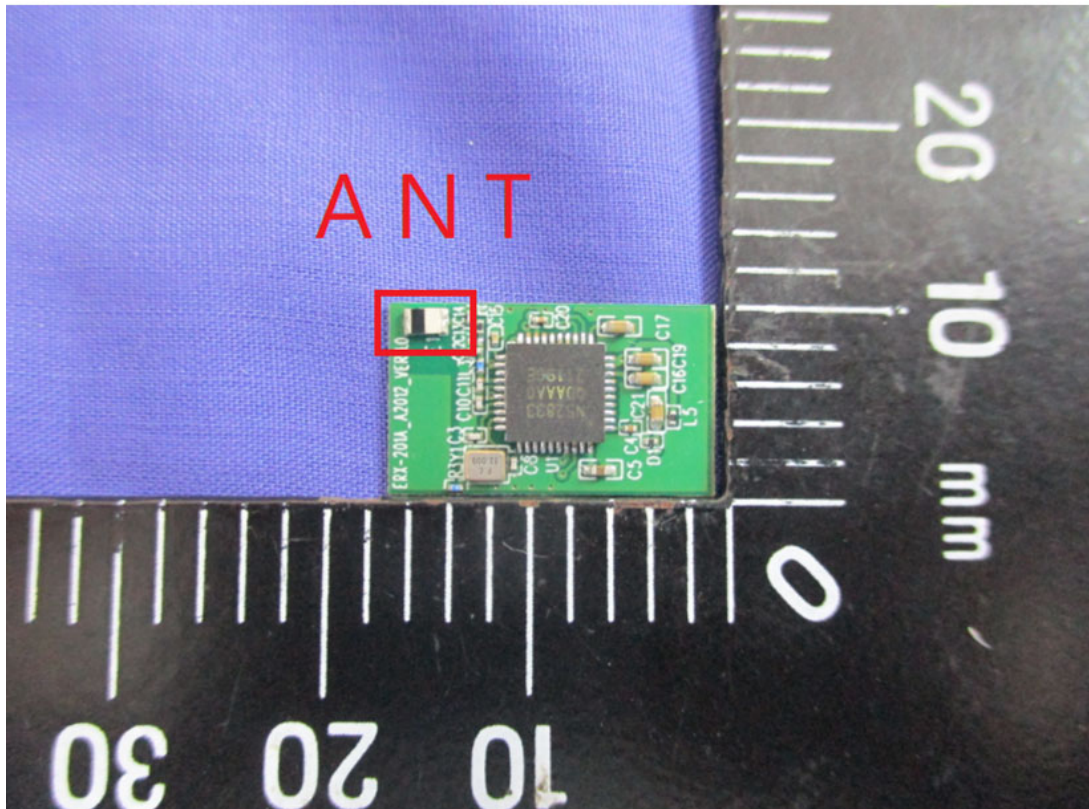
Antenna
