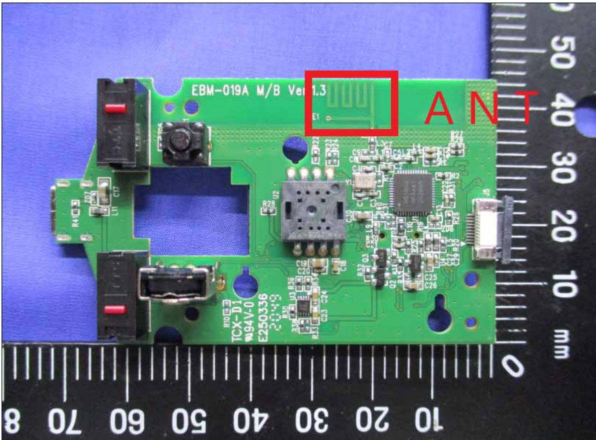
Antenna
