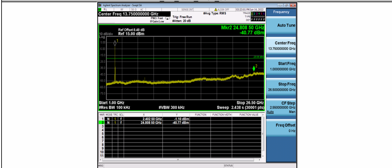
BLE 1M Ant1 2402 1000~26500
