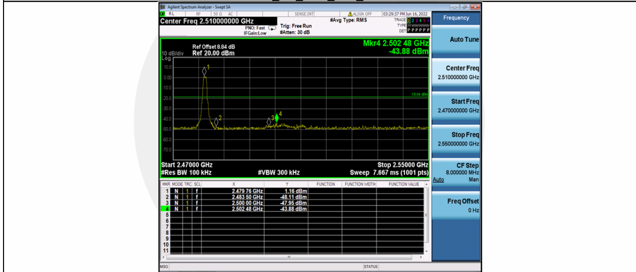
BLE 1M Ant1 High 2480
