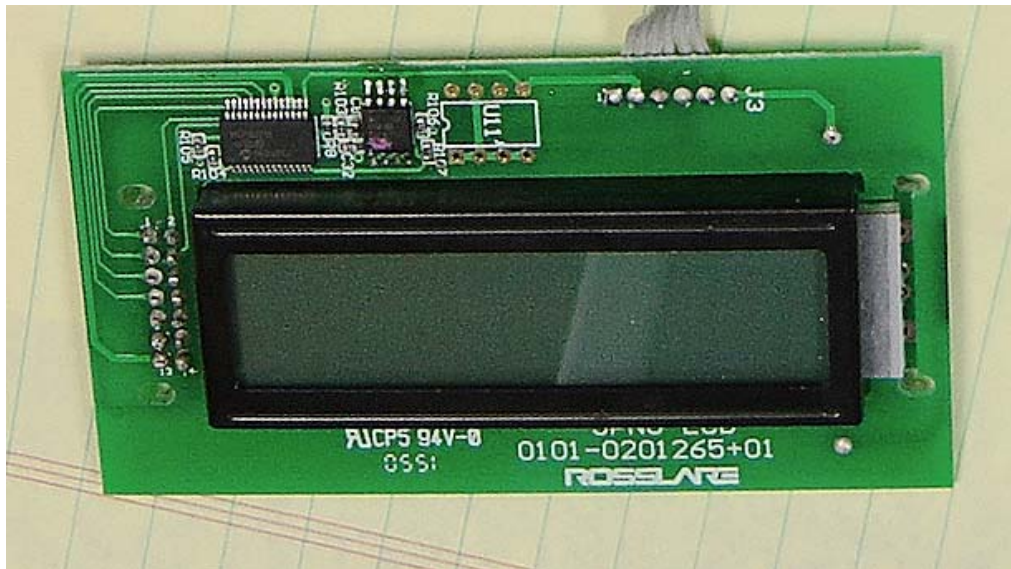
SP-N6G LCD display PCB Top
