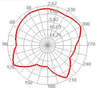
5800.000MHz E2
