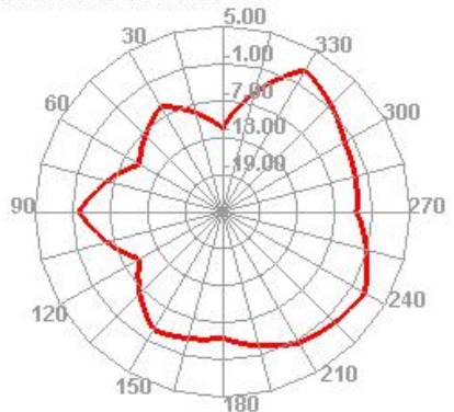
5800.000MHz H
