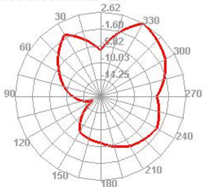
5800.000MHz E1
