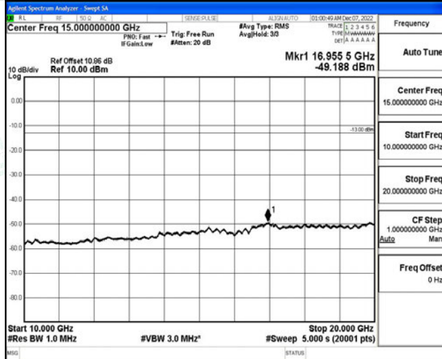
10 GHz – 20 GHz
