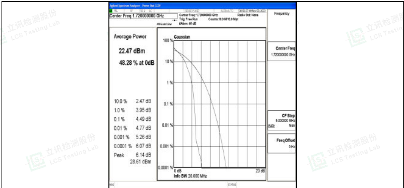
Band66-20MHz-QPSK-132072-1RB#0-PASS
