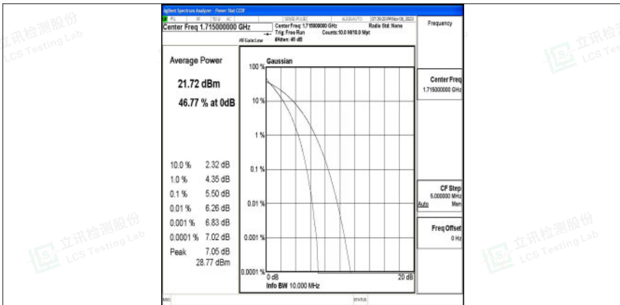
Band4-10MHz-QPSK-20000-50RB#0-PASS
