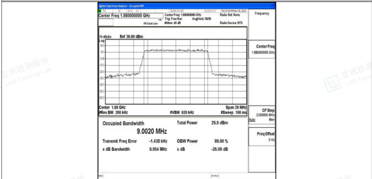
Band2-10MHz-16QAM-18900-50RB#0-PASS
