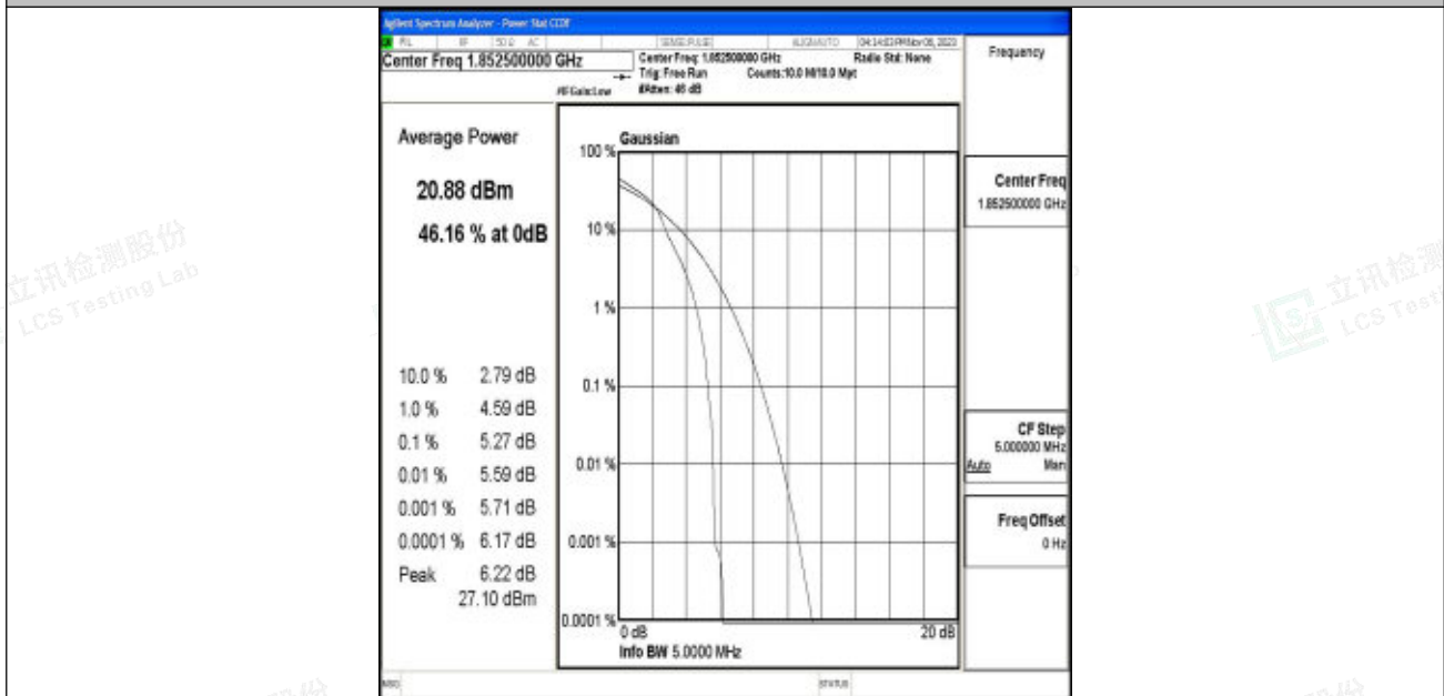
Band2-5MHz-16QAM-18625-1RB#0-PASS
