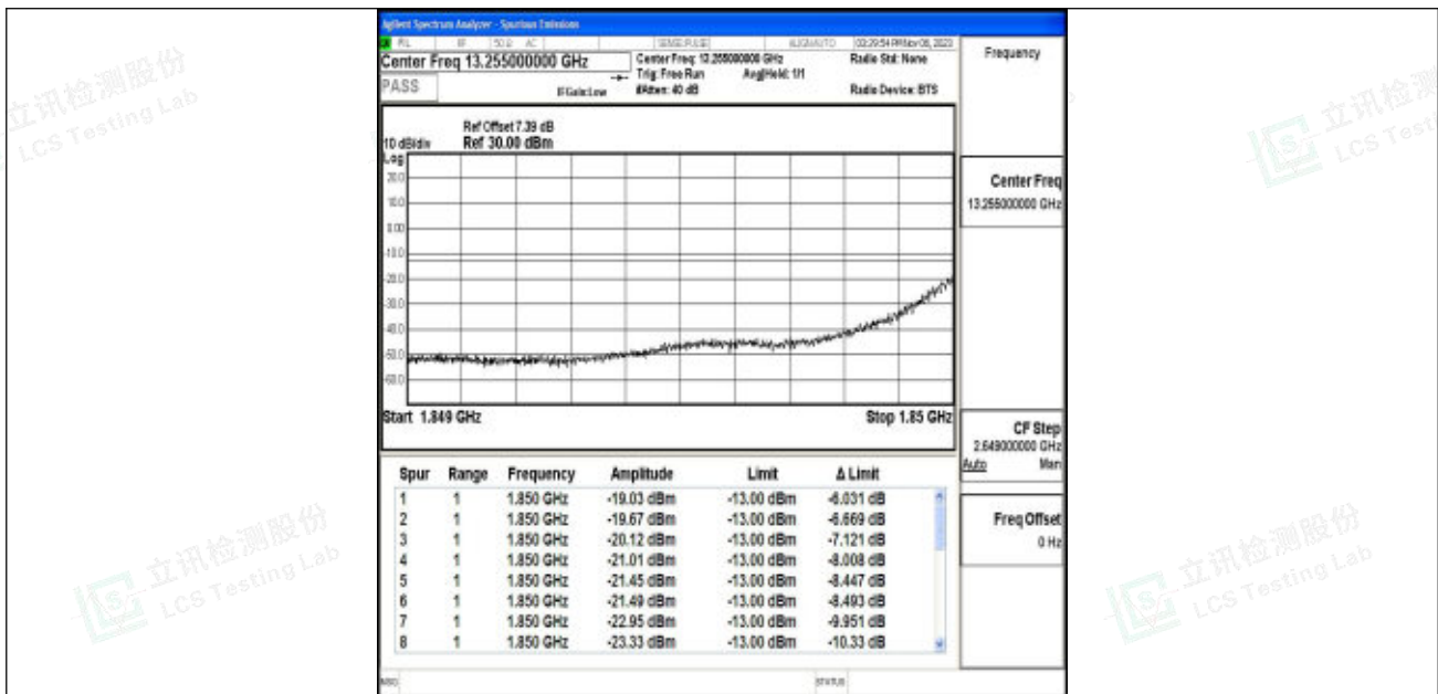
Band2_3MHz_QPSK_18615_1RB#0
