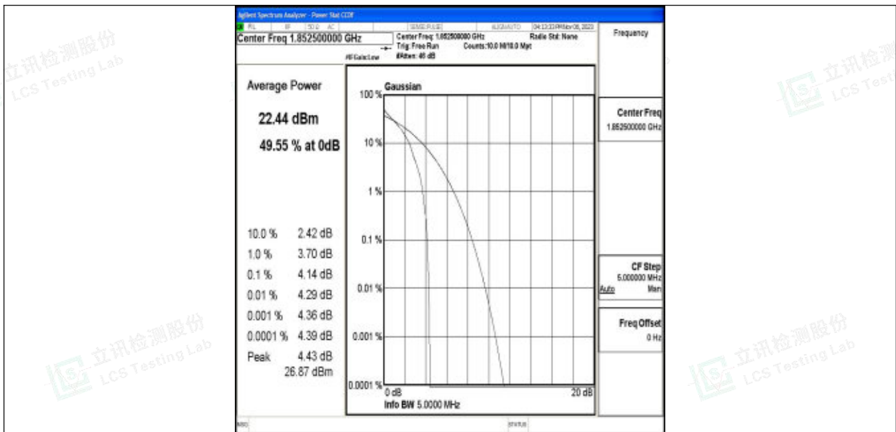
Band2-5MHz-QPSK-18625-1RB#0-PASS
