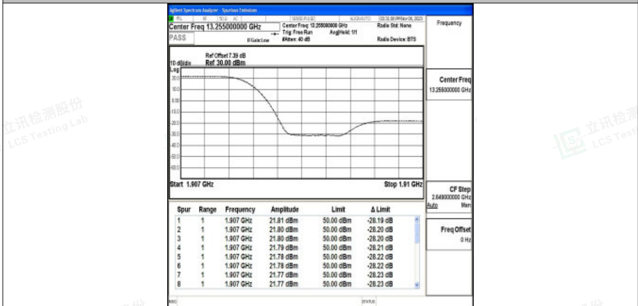
Band2_3MHz_QPSK_19185_1RB#0
