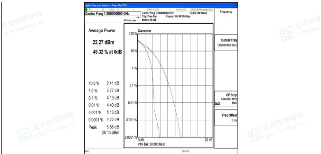
Band2-20MHz-QPSK-18700-1RB#0-PASS
