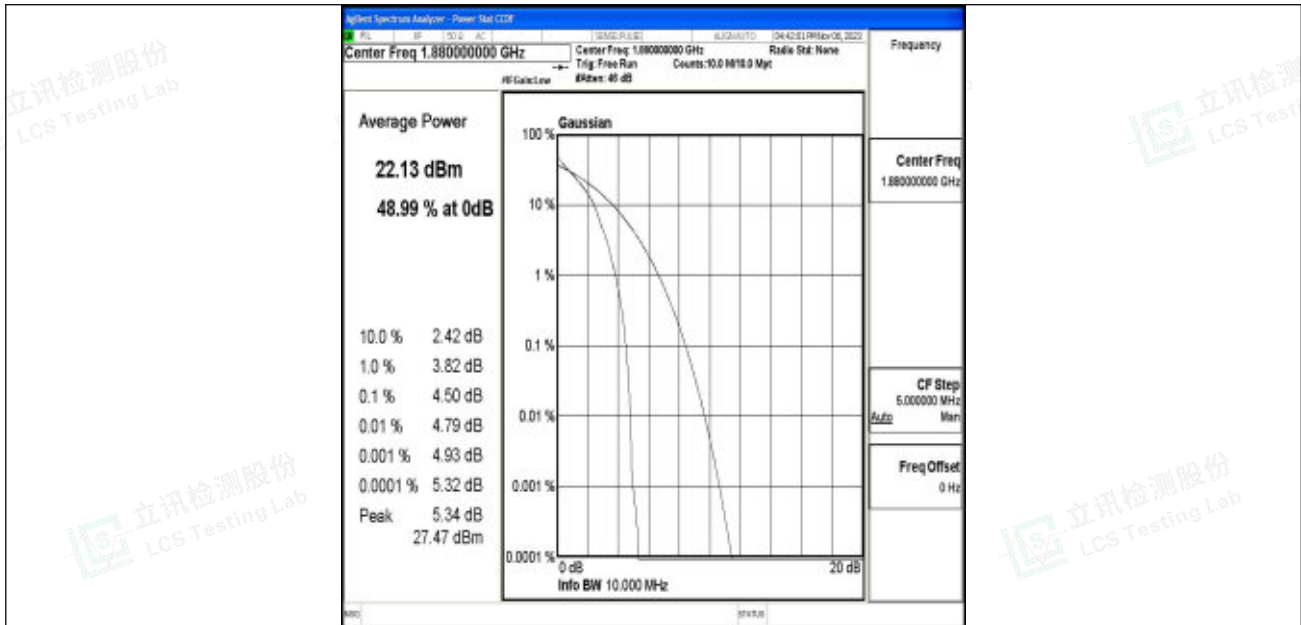
Band2-10MHz-QPSK-18900-1RB#0-PASS
