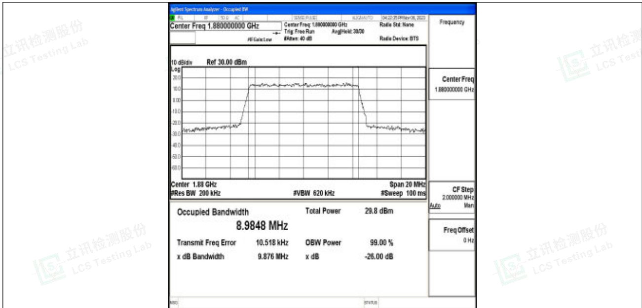
Band2-10MHz-QPSK-18900-50RB#0-PASS
