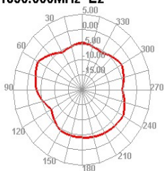
1850.000MHz E2
