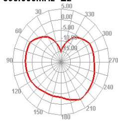
890.000MHz E2
