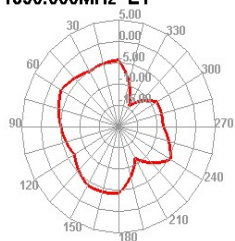
1850.000MHz E1
