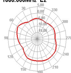
1880.000MHz E2
