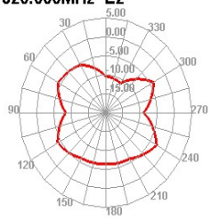
820.000MHz E2
