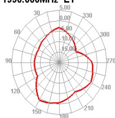
1990.000MHz E1
