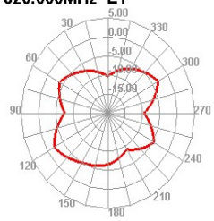
820.000MHz E1
