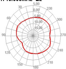
1710.000MHz E2
