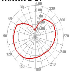
890.000MHz E1
