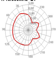
1710.000MHz E1
