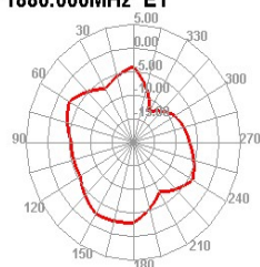
1880.000MHz E1
