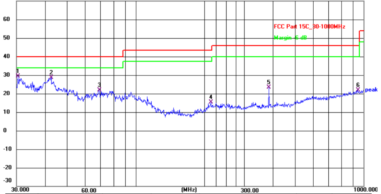
Horizontal 70.0 dBuV/m
