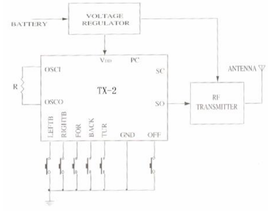
发射板流程图
