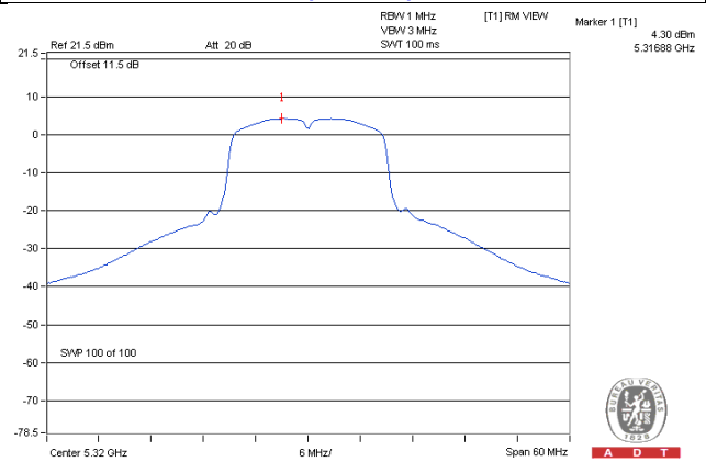
802.11n (20MHz) / CH64
