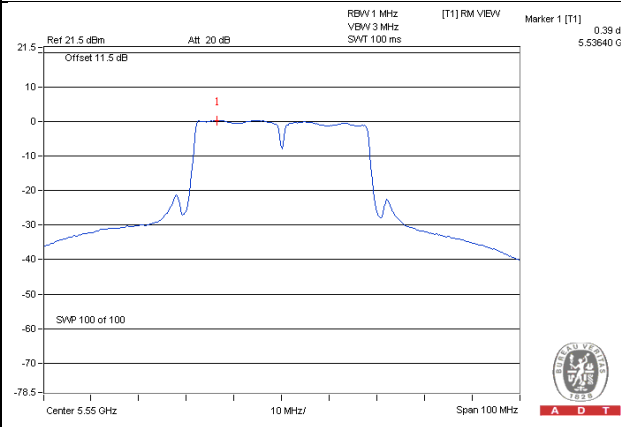
802.11n (40MHz) / CH110
