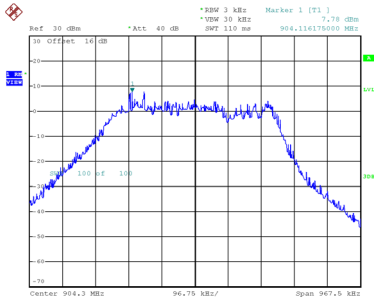
904.3MHz
