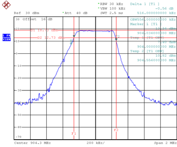
904.3MHz
