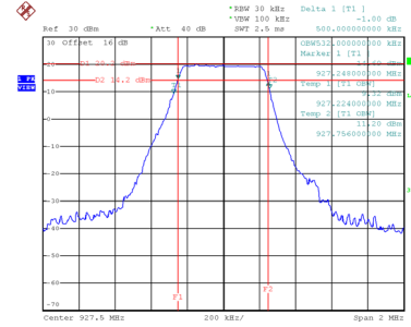
927.5MHz
