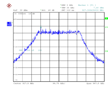
927.5MHz
