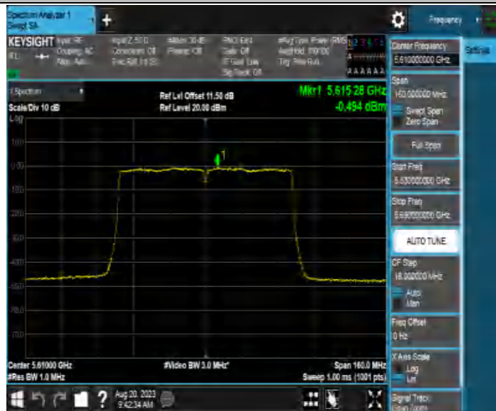
11AC80MIMO_Ant3_5610
