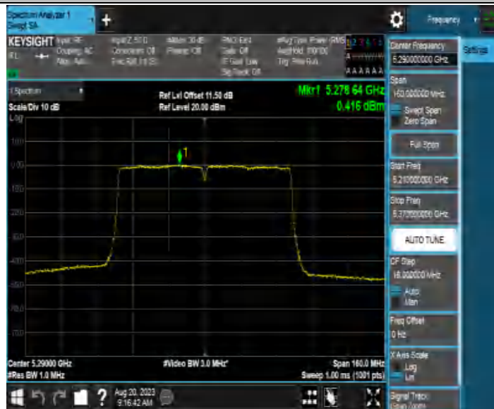
11AC80MIMO_Ant3_5290
