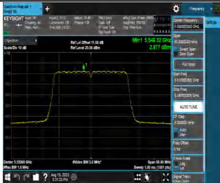
11AC40MIMO_Ant4_5550
