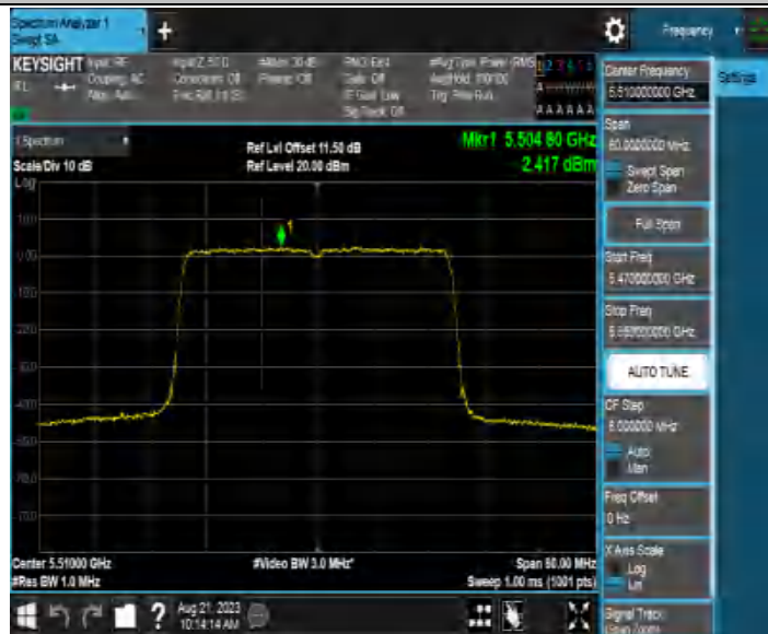
11AX40MIMO_Ant3_5510
