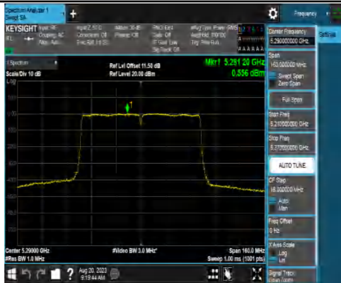
11AC80MIMO_Ant4_5290
