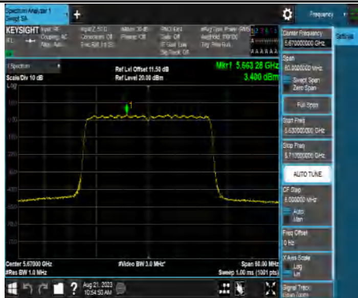
11AX40MIMO_Ant4_5670
