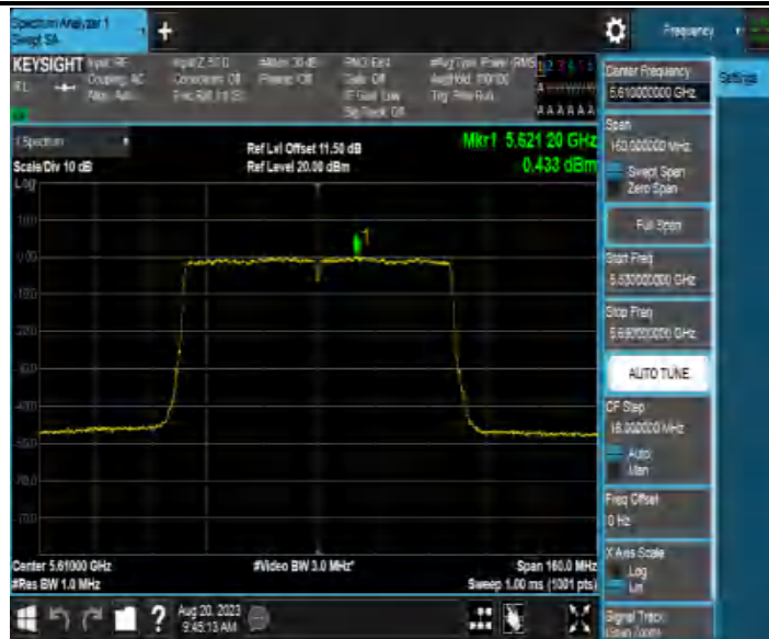
11AC80MIMO_Ant4_5610
