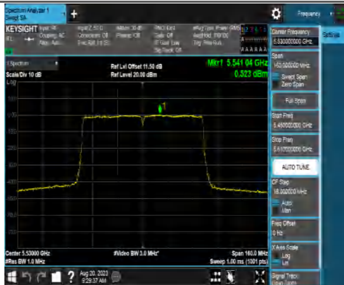
11AC80MIMO_Ant3_5530
