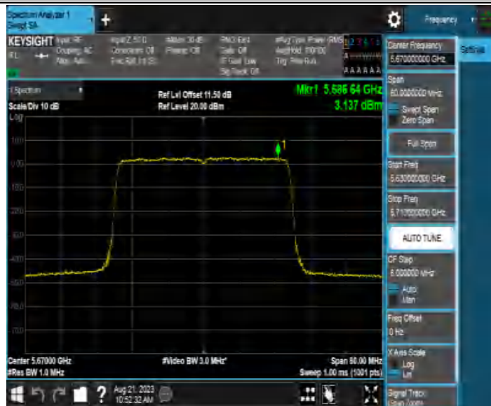
11AX40MIMO_Ant3_5670
