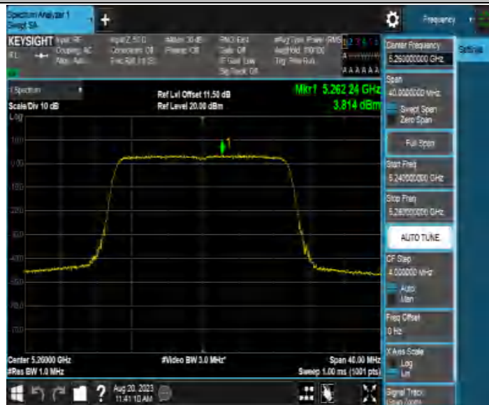
11AX20MIMO_Ant3_5260
