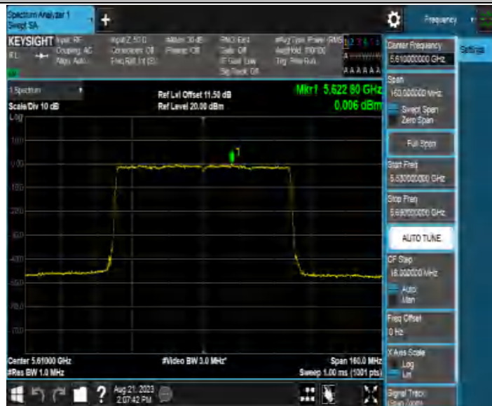
11AX80MIMO_Ant3_5610
