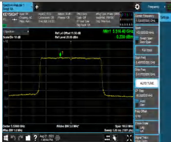
11AX80MIMO_Ant3_5530
