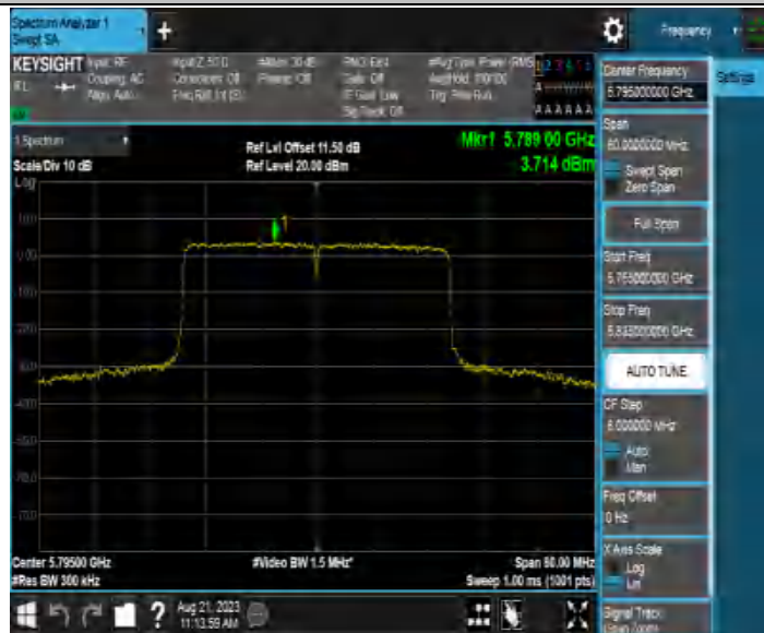
11AX40MIMO_Ant3_5795
