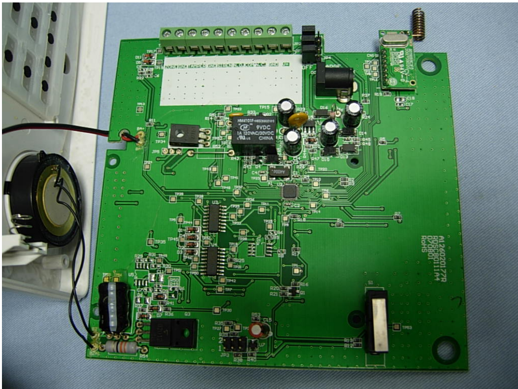
(10) EUT Photo (Host-M/N: SC801-2)
