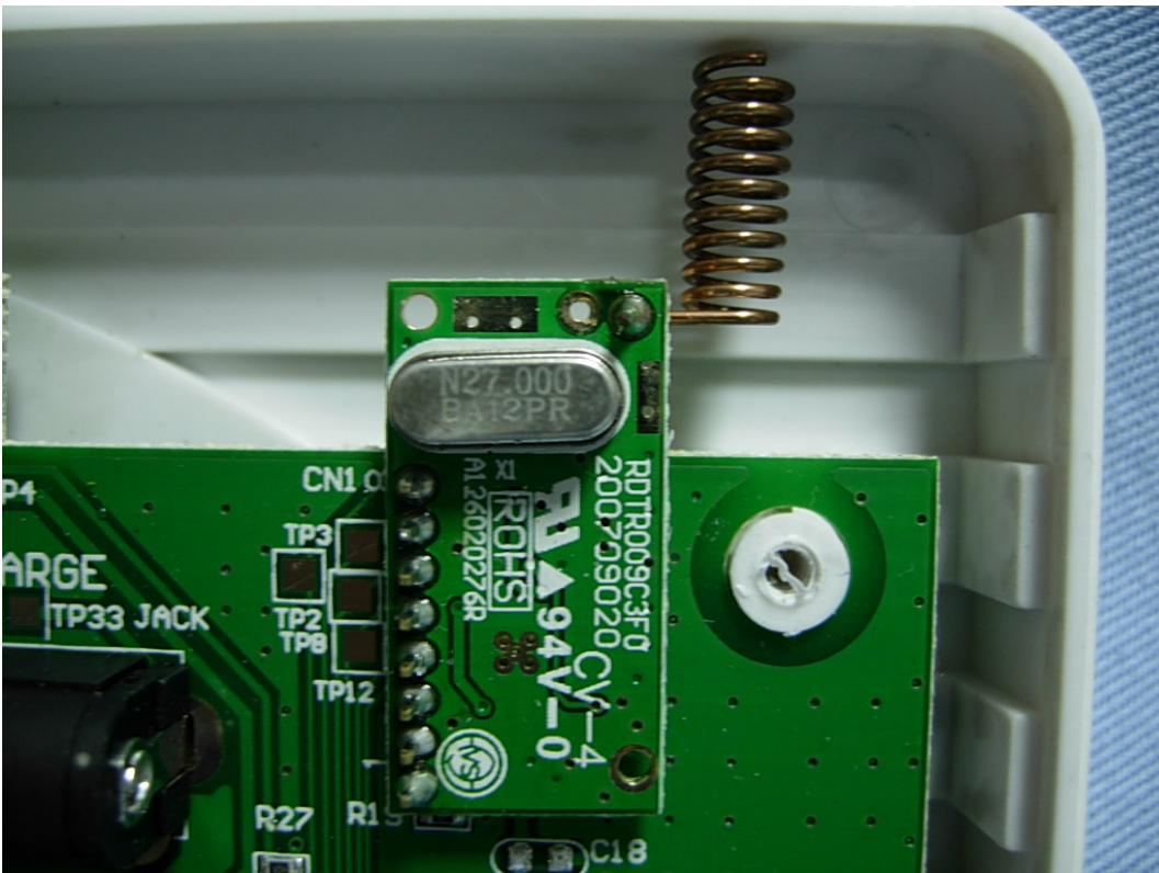
(8) EUT Photo (Host-M/N: SC801-2)
