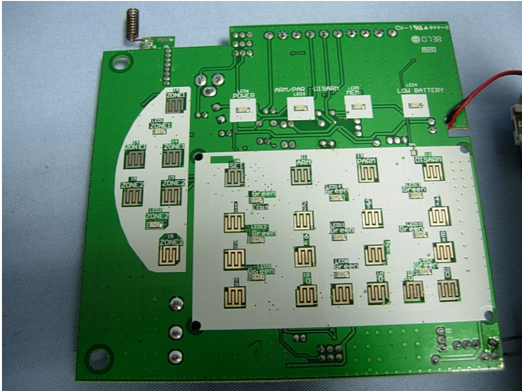
(9) EUT Photo (Host-M/N: SC801-2)
