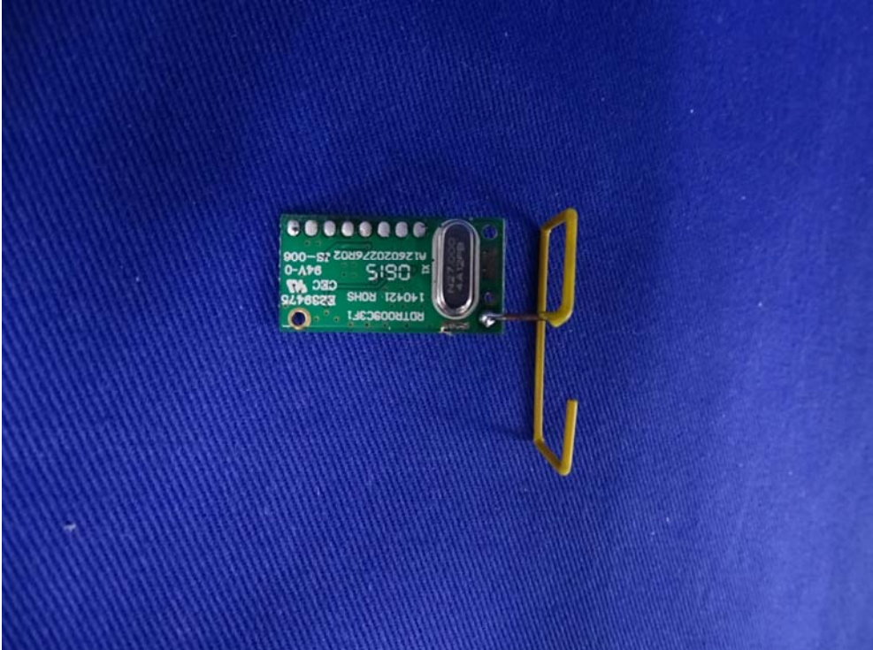
(16) EUT Photo
