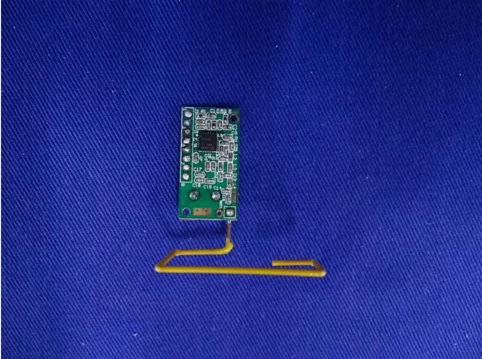
(15) EUT Photo
