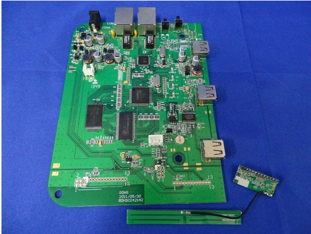
(26) EUT Photo - Z-wave module
