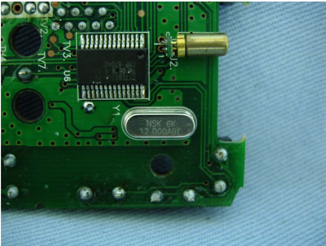
(9) EUT Photo
