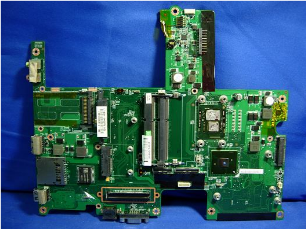
(84) EUT Photo
