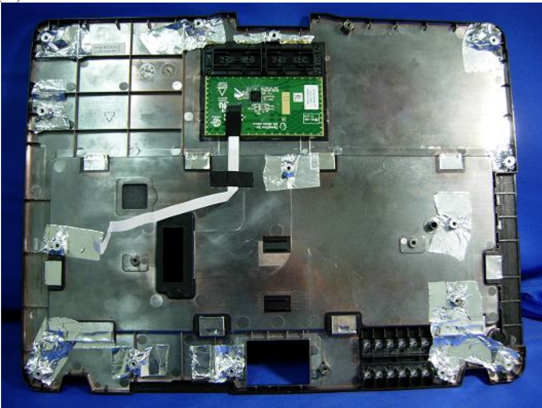
(58) EUT Photo
