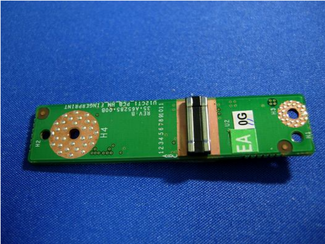
(94) EUT Photo
