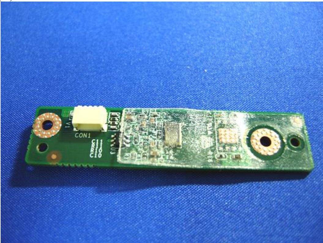
(94) EUT Photo
