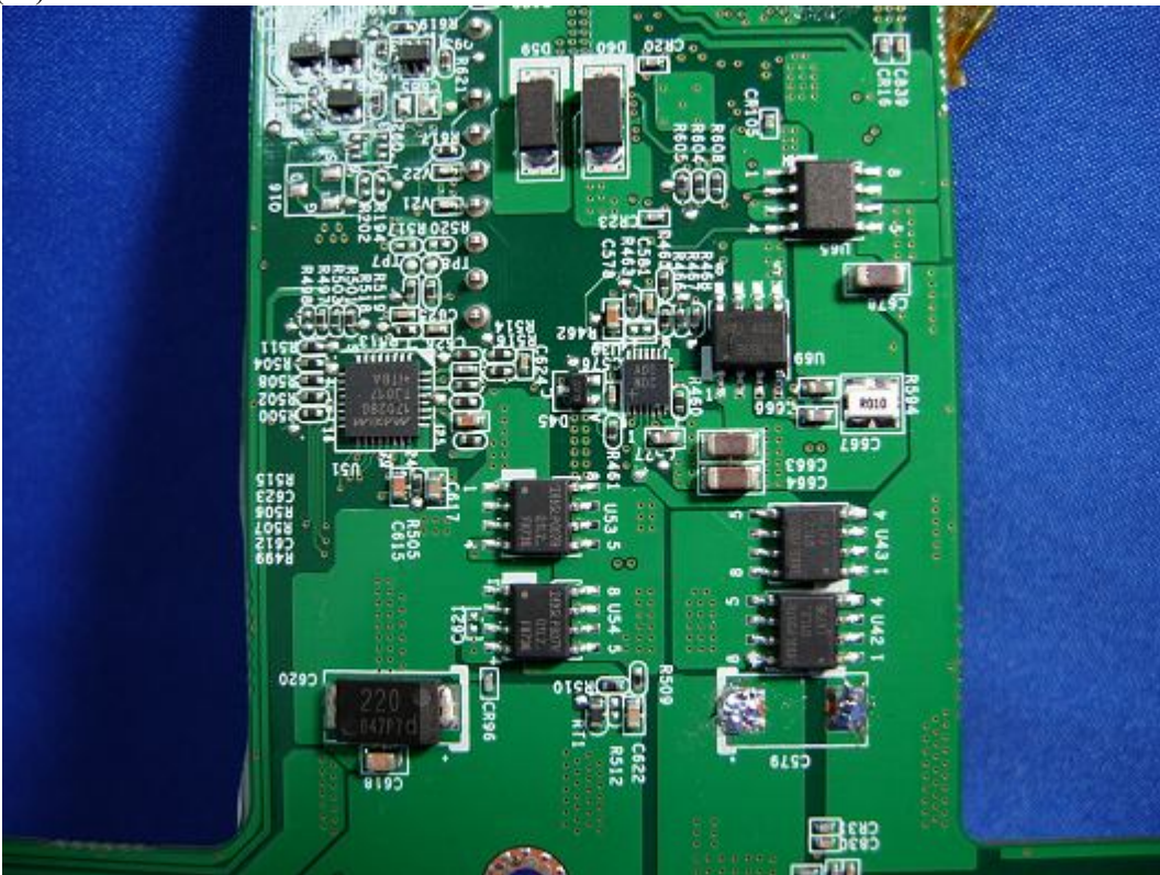
(74) EUT Photo
