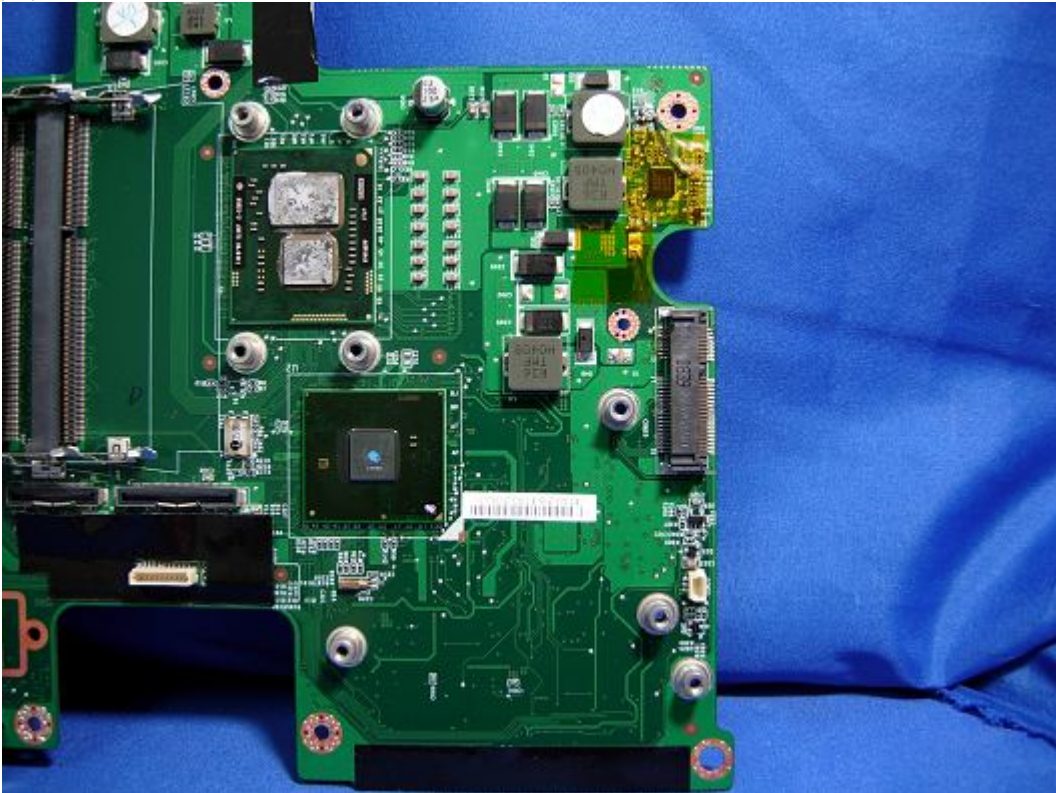
(88) EUT Photo
