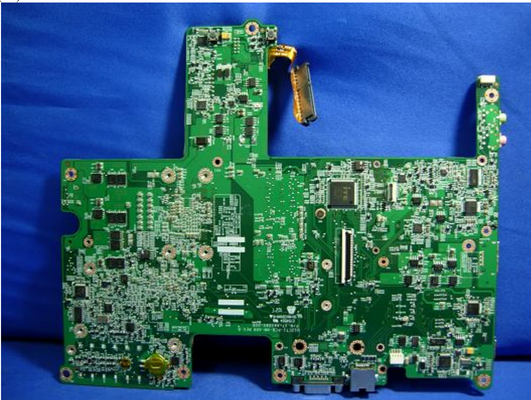
(72) EUT Photo
