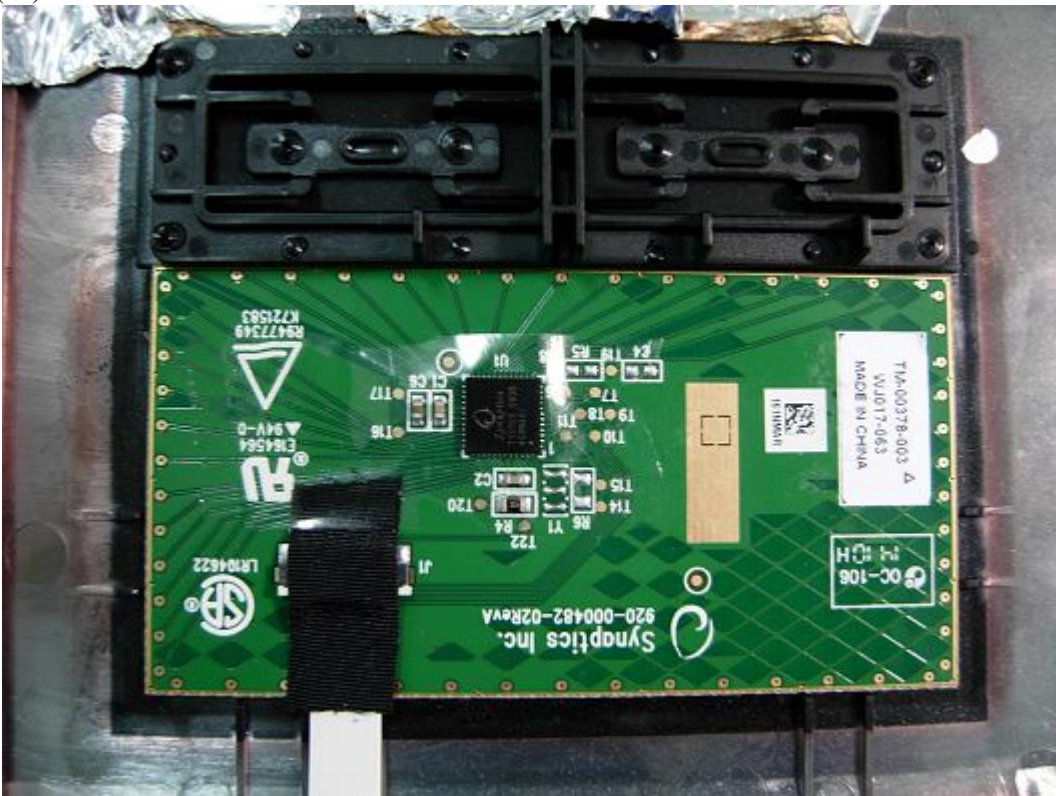
(60) EUT Photo
