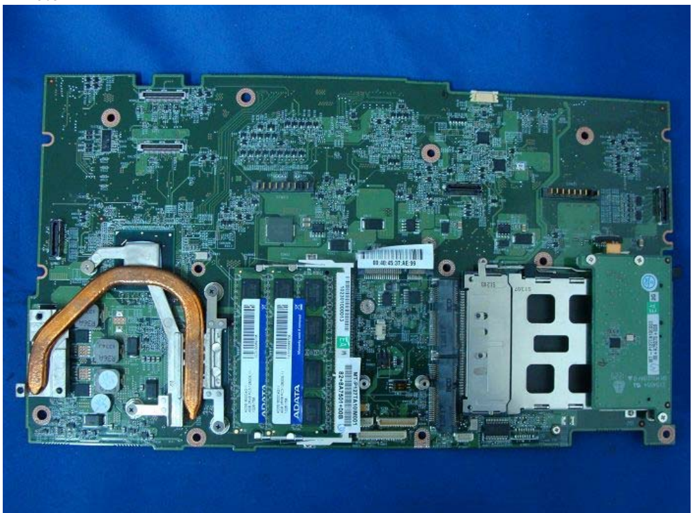
(30) EUT Photo
