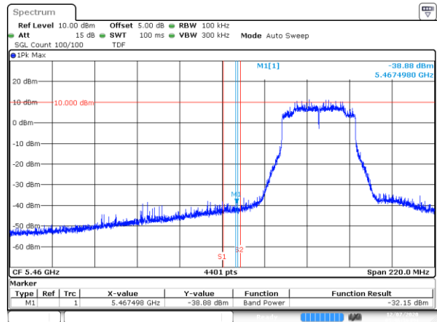
BE-NR-LOW, SISO-A, 802.11ax40-HE0, Ch102
