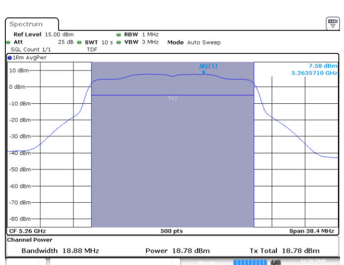
MIMO B-802.11ax-20MHz-Ch52-5260MHz-HE0
