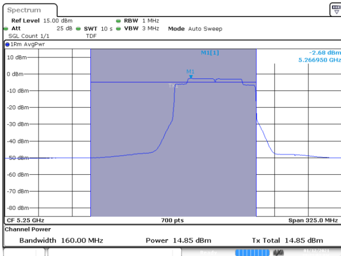
MIMO A-802.11ax-160MHz-Ch50-5250MHz-HE0-996/S67
