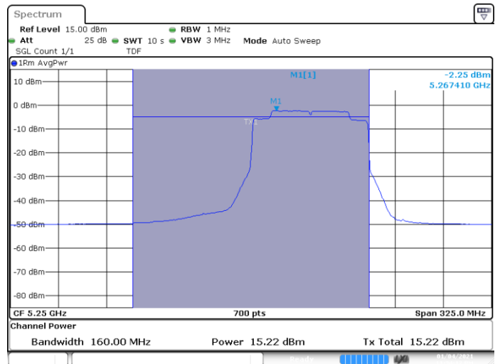
MIMO B-802.11ax-160MHz-Ch50-5250MHz-HE0-996/S67
