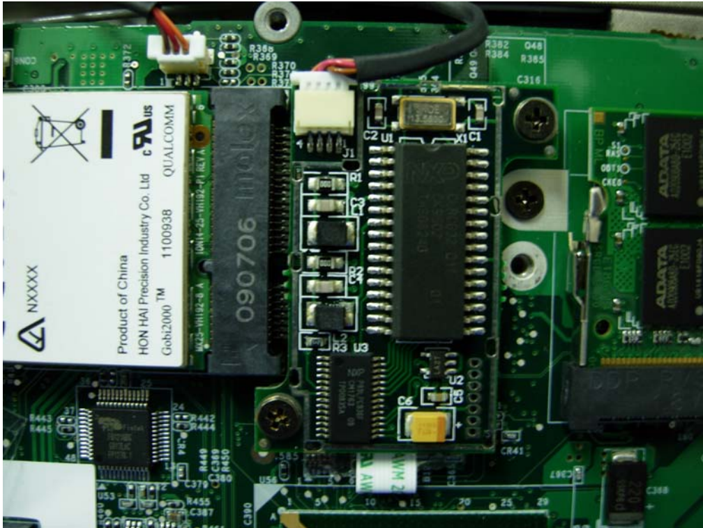
(15) EUT Photo - (RFID Module)
