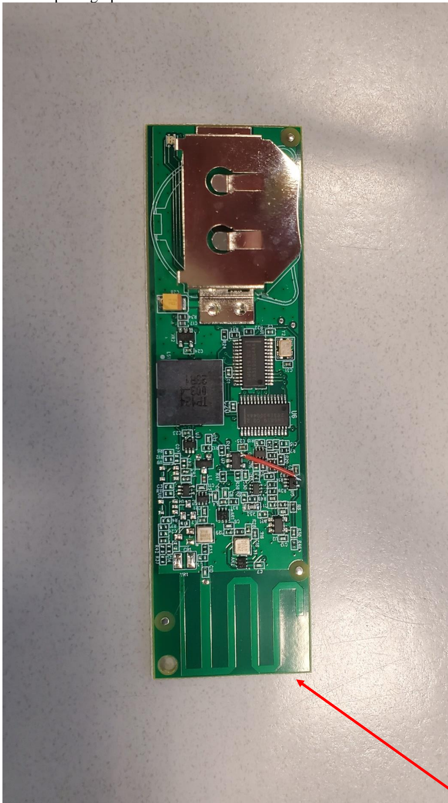
Antenna
