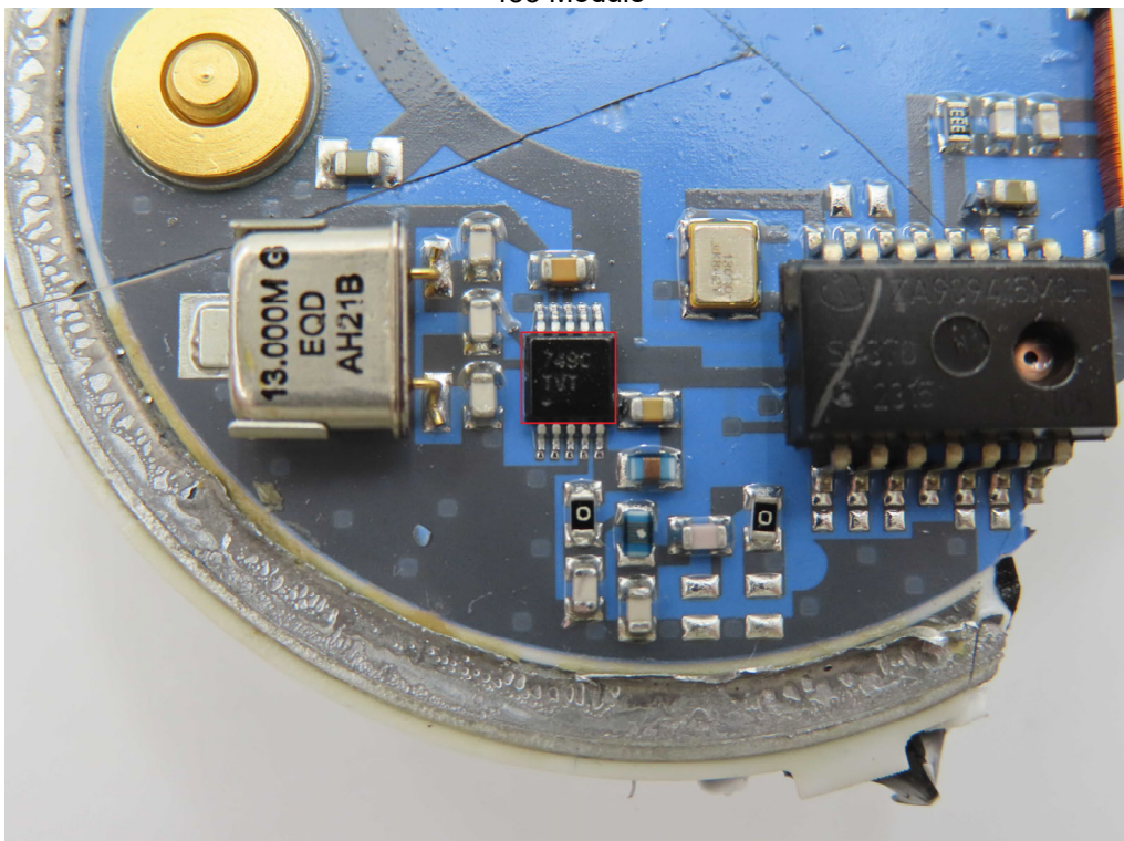
433 Module
