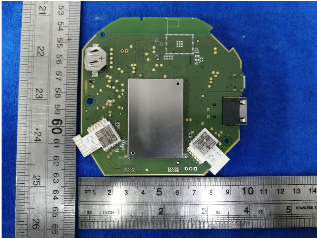
Bild / Picture 2: Mainboard PCB
