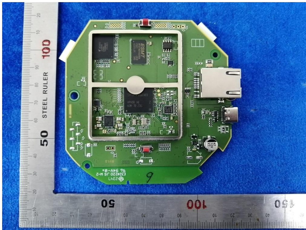
Bild / Picture 4: Mainboard PCB
