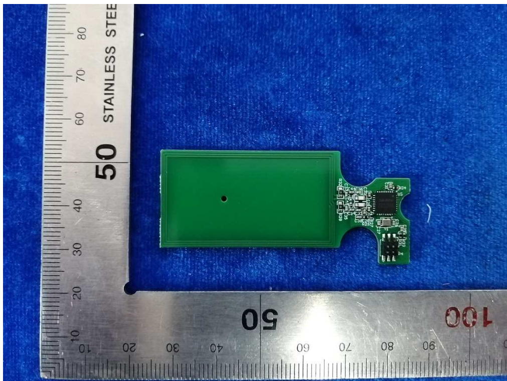
Bild / Picture 6: NFC PCB
