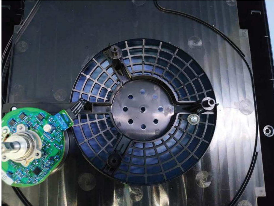
Fan motor brackt and fan guard
