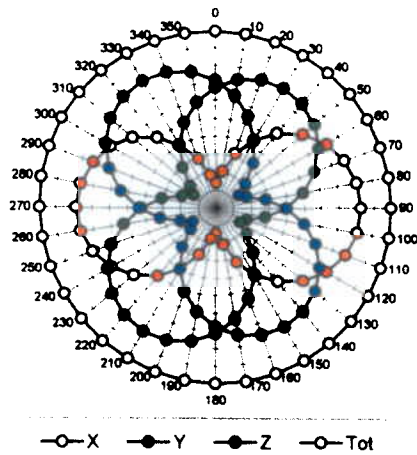
f = 30 MHz, TEM cell I#110
