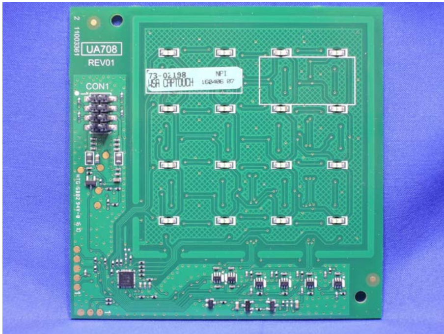
(18) EUT Photo
