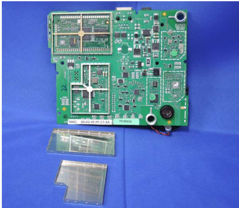
(20) EUT Photo
