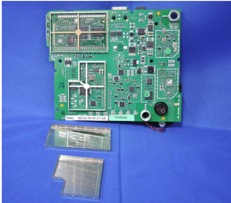
(19) EUT Photo
